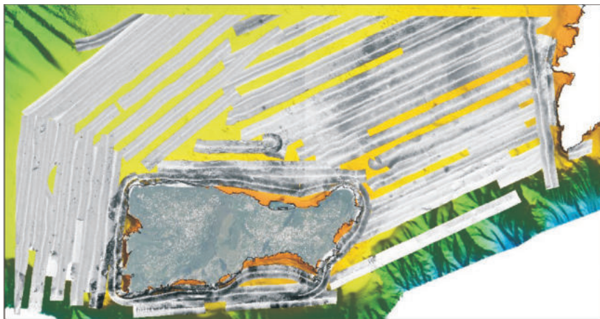
Fig. 3 - Copertura delle indagini Sidescan sonar.
