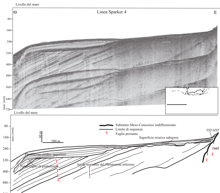
Fig. 20 - Linea Sparker 4 (ubicazione nel riquadro) del margine continentale nel tratto occidentale del foglio. Sono visibili la dislocazione in profondità del substrato carbonatico ed i set di sequenze del Pleistocene inferiore e medio.
